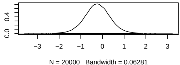
Density of d.Placebo.Erlotinib
